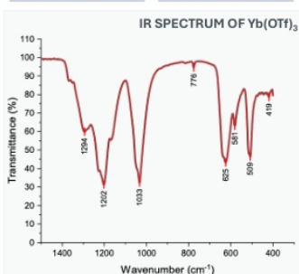
Fig. 3 IR spectrum of Yb(OTf) 3
